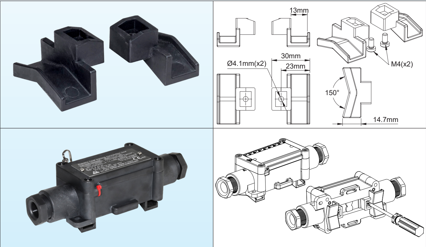
Y40伴热接线盒的组装示例
