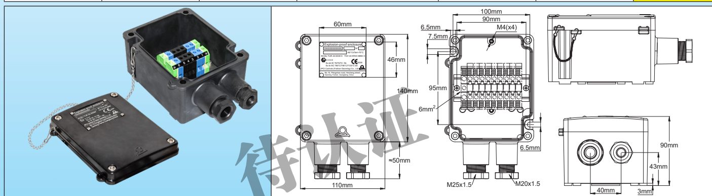
带接线柱的示例
