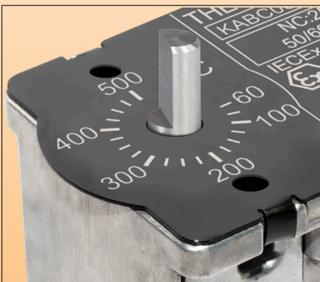
A: 轴直径6mm，长度10mm，用于印刷旋钮和边框，或小塑料箭头旋钮 (可作为下面的配件提供);
