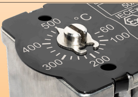
C: 螺丝刀的型号，带箭头和印刷的铝表盘，用于 JPCI 或其他供应商的 PPS Ex-e 外壳进行伴热；
